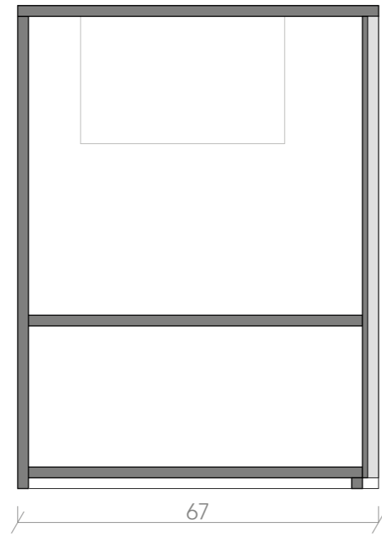
Coupe BB
